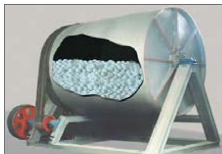
شکل ۲۴ - آسیاب گلوله‌ای
