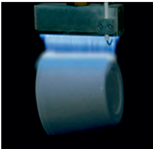
شکل های ۴۵-۳ روش شعله زنی
