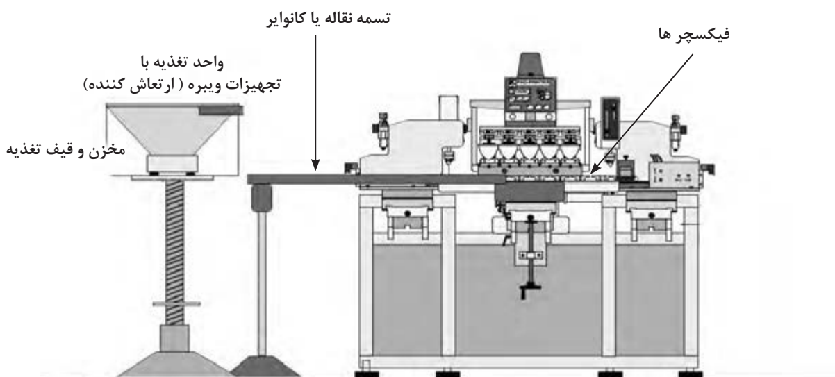
شکل ۶۲-۳ نمای شماتیک تغذیه خودکار
