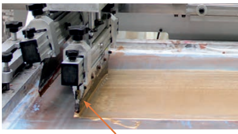
شکل ۵-۱۱ ایجاد پله در نقطه شروع حرکت اسکوئیجی
