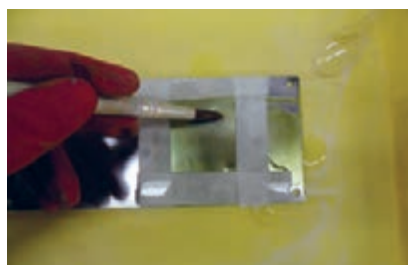
شکل ۴-۲۴- اسیدکاری کلیشه
