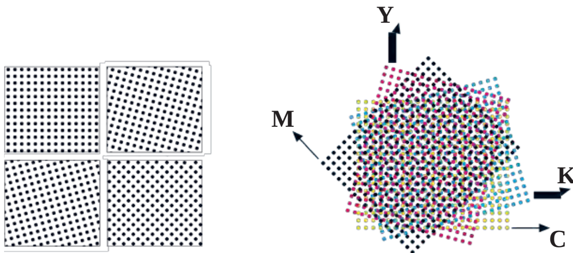
شکل ۸-۳- زوایای ترام
