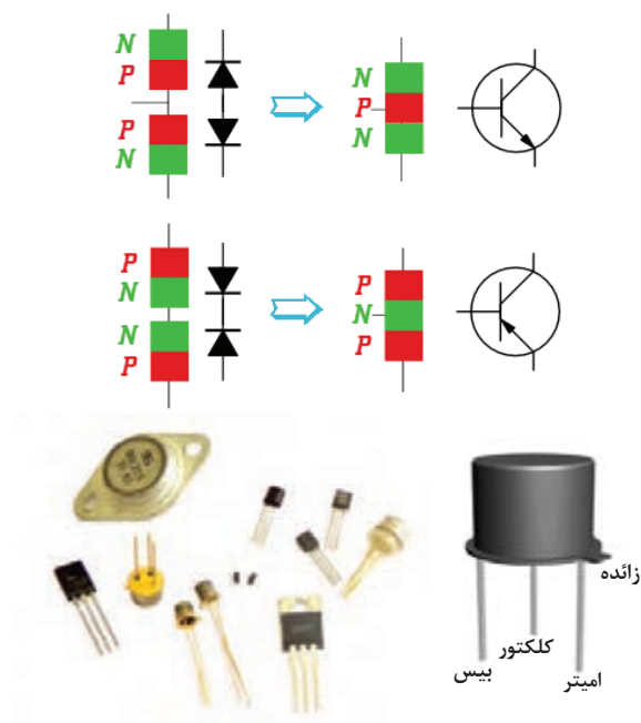
شکل ۱۸-۱ ترانزیستور
